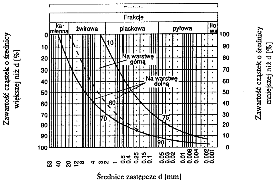
Rys. 2. Obszar uziarnienia optymalnej mieszanki gliniasto-żwirowej
